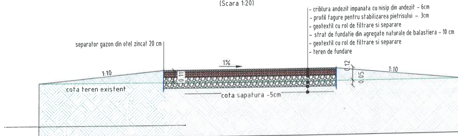
Detaliu 2 Structura alei secundare si alveole secundare (Scara 1:20)
