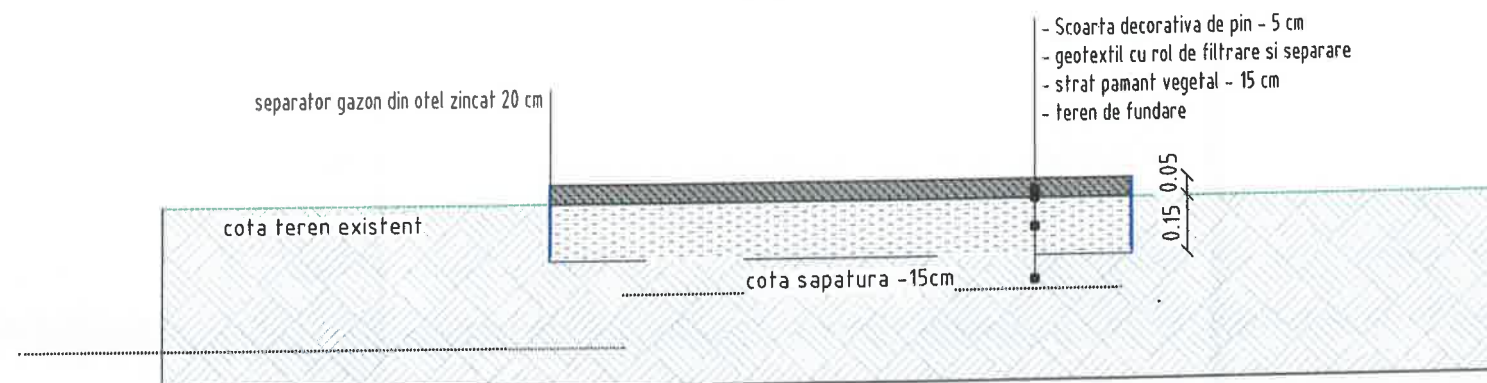
Detaliu 3 Structura zone plantare plante perene (Scara 1:20)
