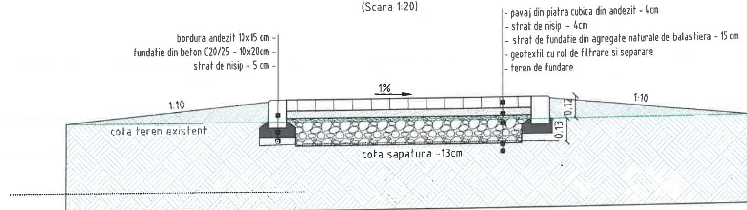
Detaliu 1 Structura alei principale (Scara 1:20)
