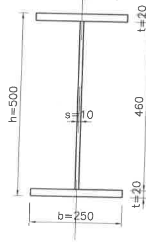
DETALIU GRINDA PRINCIPALA Scara 1:10
