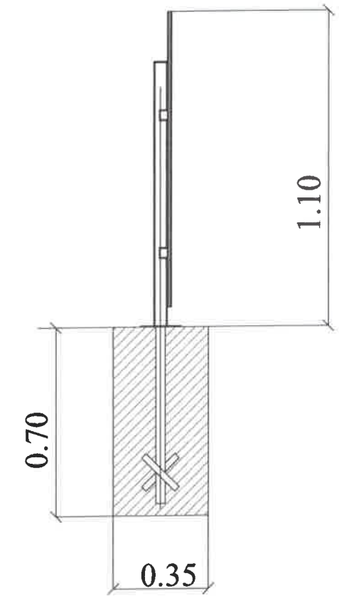
SECTIUNE 1/20
