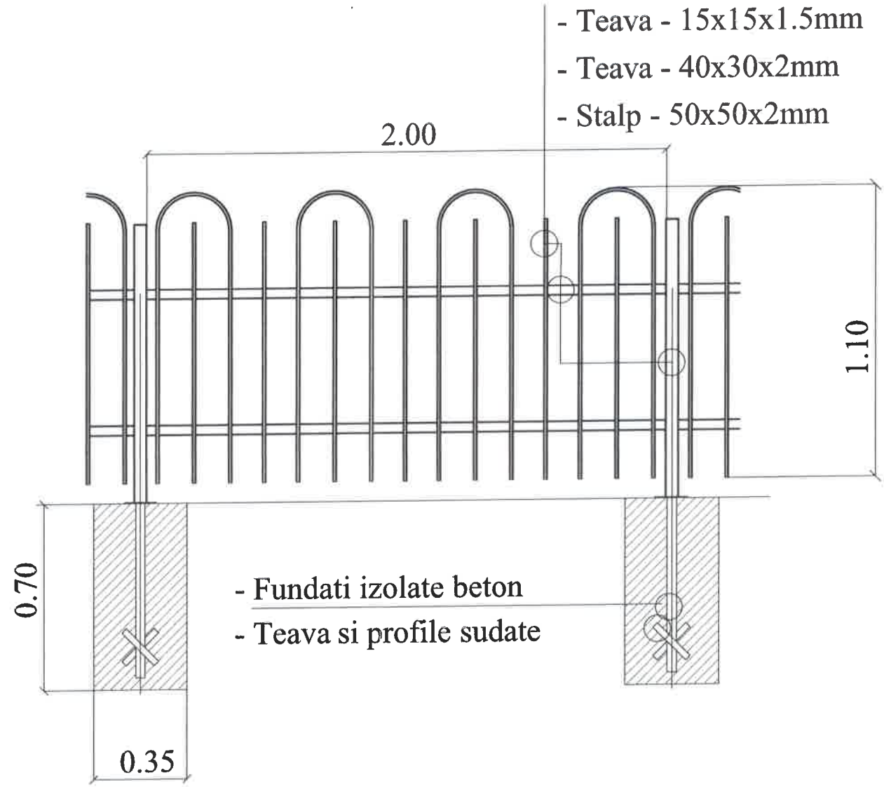
VEDERE 1/20
