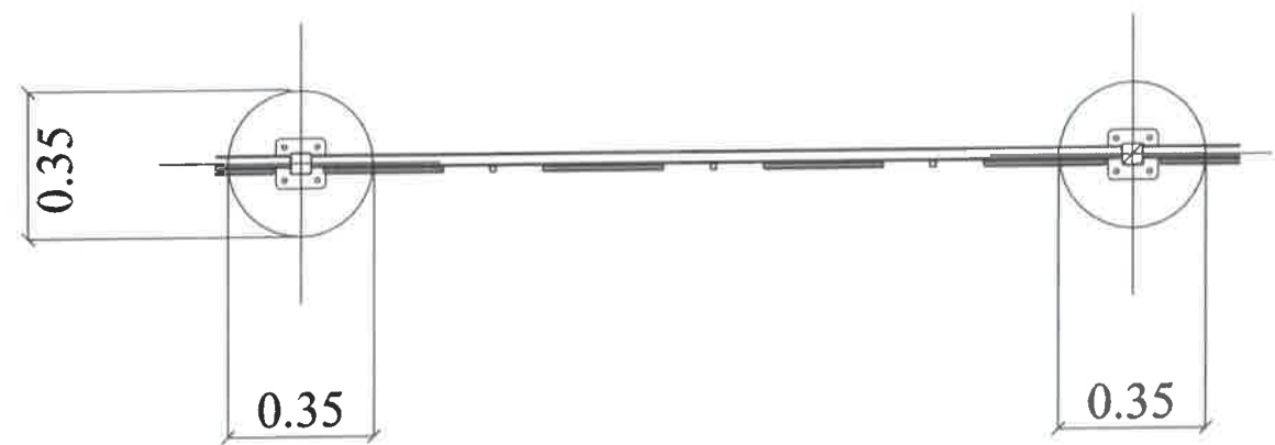
PLAN 1/20
