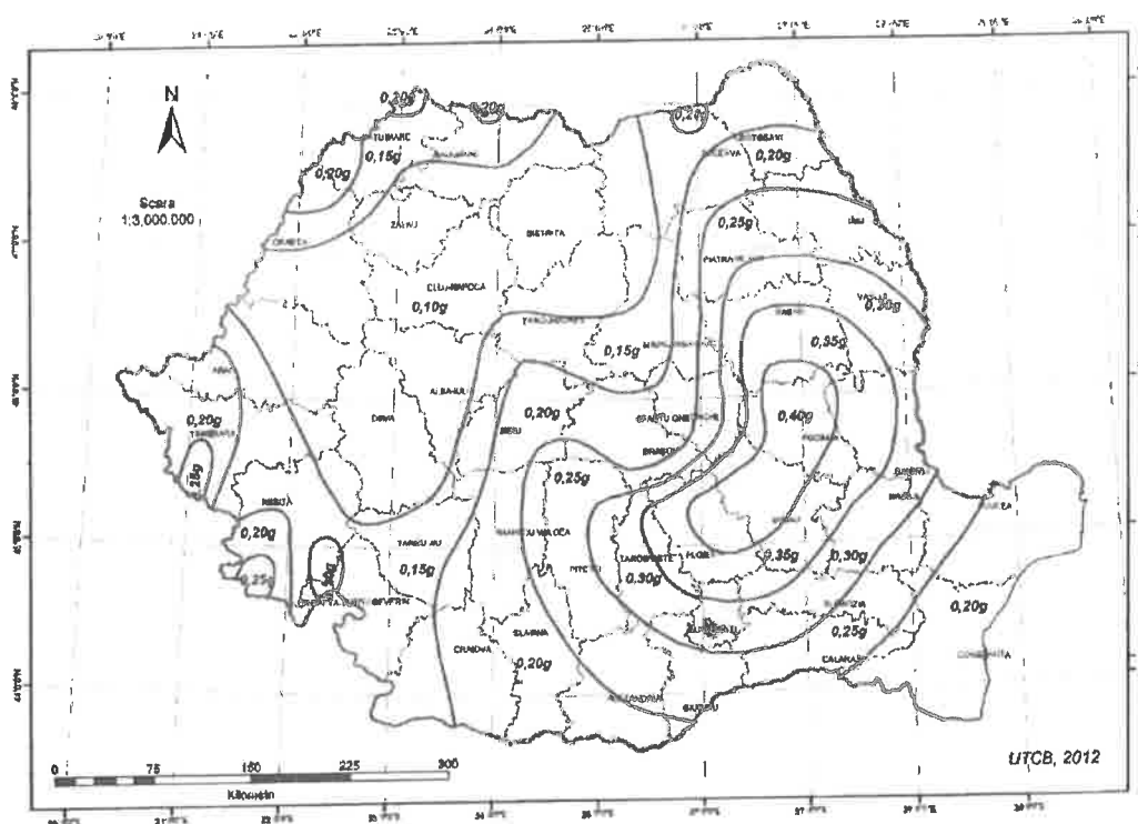
Fig. 5 Zonarea teritoriului Romaniei in termeni de valori de varf ale acceleratiei terenului pentru proiectare ag pentru cutremure avand intervalul mediu de recurenta IMR=225 ani, conform P100-1/2013 „Cod de proiectare seismica”
