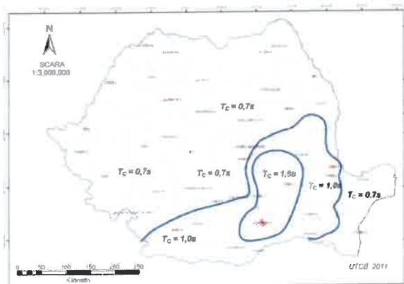
Figura A.2 Zonarea teritoriului României în termeni de perioada de control (colți), T_c a spectrului de raspas
