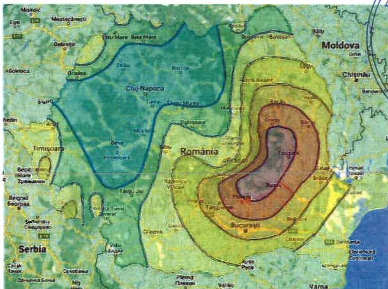
Zonarea teritoriului României în termeni de valori de vârf ale accelerației terenului de proiectare a_g pentru cutremure având intervalul mediu de recurență IMR= 225 ani și 30% probabilitate de depășire în 50 de ani
