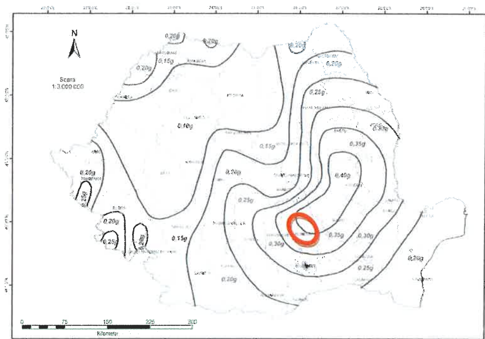
Figura 3 – Zonarea valorilor de vârf ale accelerației terenului pentru proiectare a_g = 0.25 \text{ g} cu IMR=100 ani
