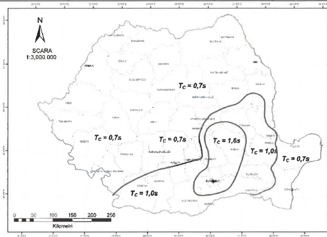
Fig. Zonarea teritoriului României în termeni de perioadă de conțon (colț), T_c a spectrului de răspuns
