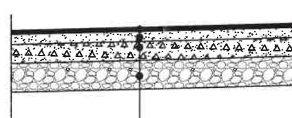
PROFIL TRANSVERSAL TIP TEREN SPORT Scara 1:50
