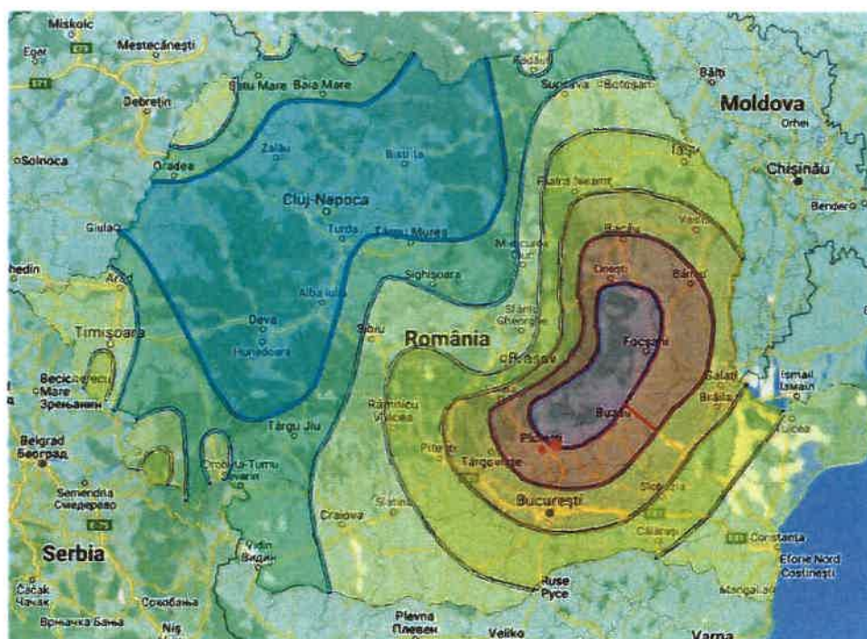
Zonarea teritoriului României în termeni de valori de vârf ale accelerației terenului de proiectare a_g pentru cutremure având intervalul mediu de recurență IMR= 225 ani și 20% probabilitate de depășire în 50 de ani
