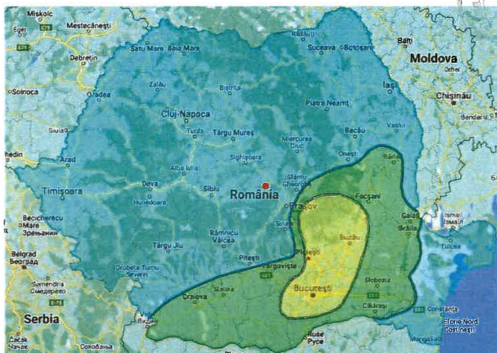
Zona teritoriului României în termeni de perioadă de control (colt), T_c a spectrului de răspuns
