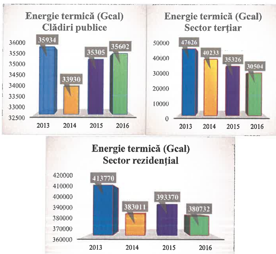
Figura 13 Energia termică distribuită consumatorilor din municipiul Ploiești
