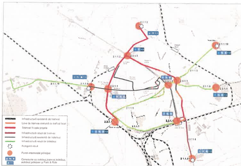
Figura 10 Măsuri de infrastructură propuse pentru transportul public
