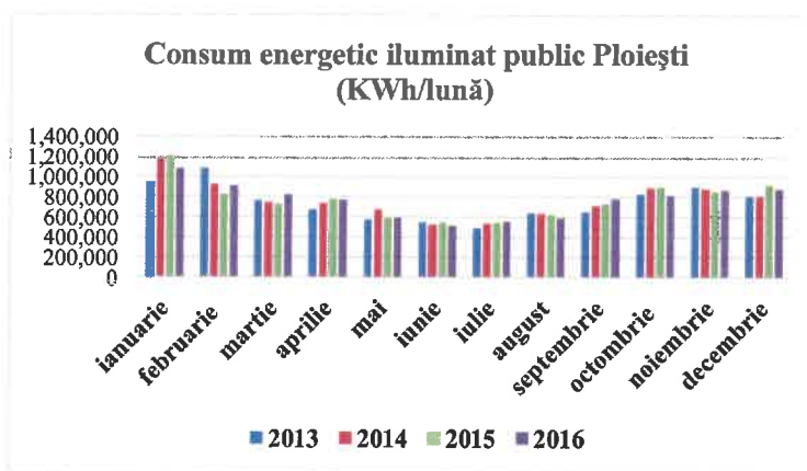
Figura 28 Evoluția consumurilor lunare în perioada 2013-2016 Sursa: date Municipiul Ploiești
