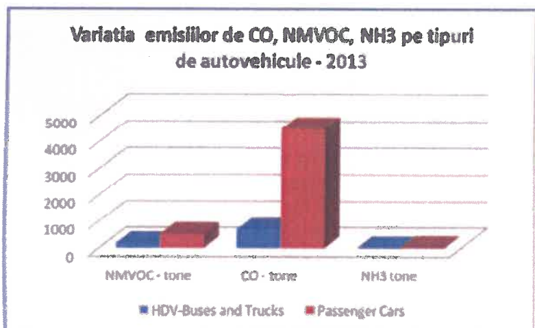
Figura 16 Variația emisiilor/ tipuri de autovehicule în anul 2013 - municipiul Ploiești Sursa: PMUD
