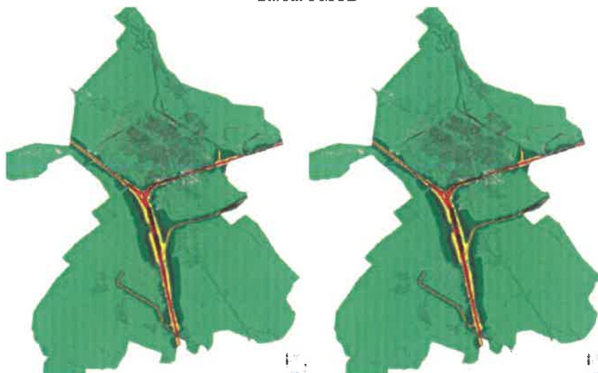
Figura 20 Aglomerarea urbană Ploiești - sursa căi ferate tren, indicatorul Lzsn (stânga) și Lnoapte (dreapta)
