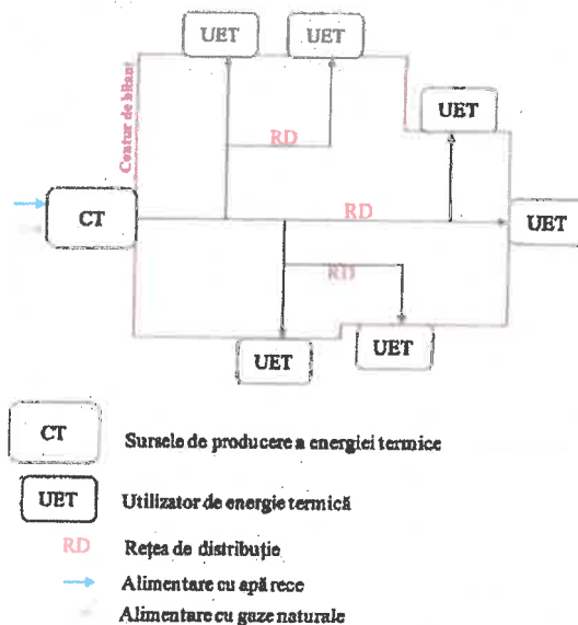
Figura 5.2 – Schema fluxului tehnologic din conturul de bilanț al RD aferentă CT de cvartal
