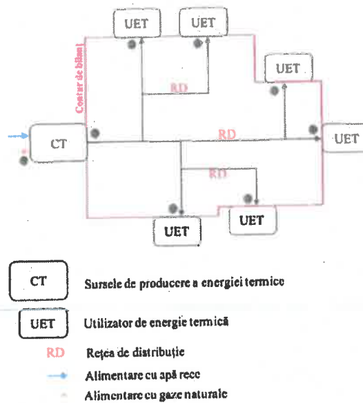
Figura 9.2 – Schema fluxului tehnologic din conturul de bilanț al RD aferentă CT de cvartal, cu punctele de măsură
