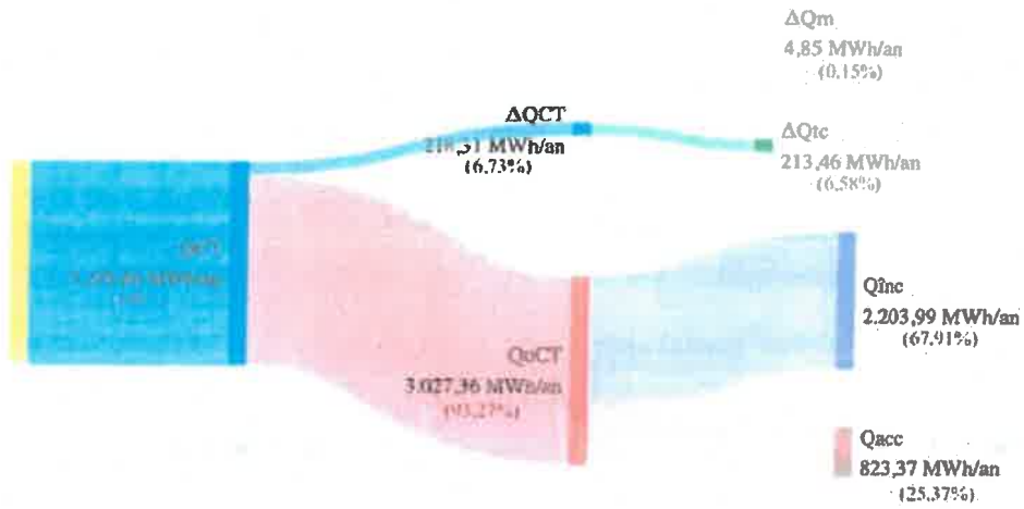
Figura 17.3 – Diagrama Sankey pentru regimul optimizat de funcționare a RD aferentă CT
