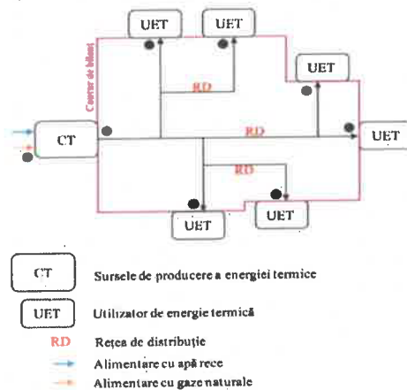
Figura 2 – Schema fluxului tehnologic din conturul de bilanț al RD aferentă CT de cvartal, cu punctele de măsură
