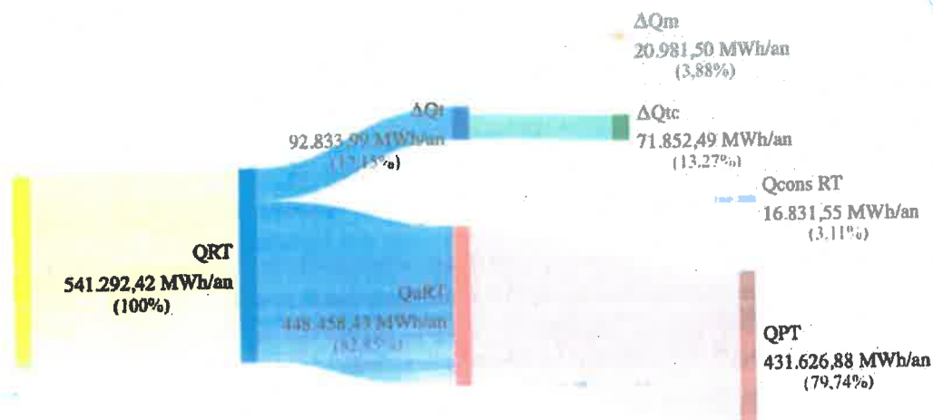
Figura 17.1 – Diagrama Sankey pentru regimul optimizat de funcționare a RT
