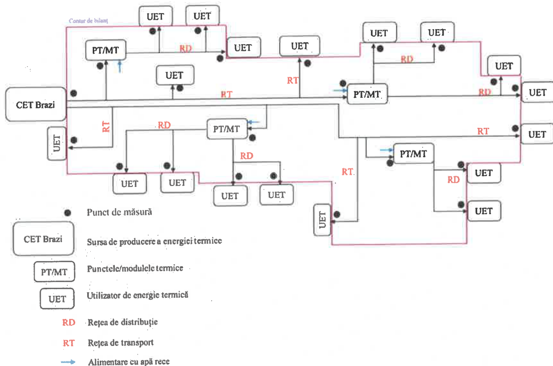
Figura 1 – Schema fluxului tehnologic din conturul de bilanț al RT și RD aferente PT/MT, cu punctele de măsură
