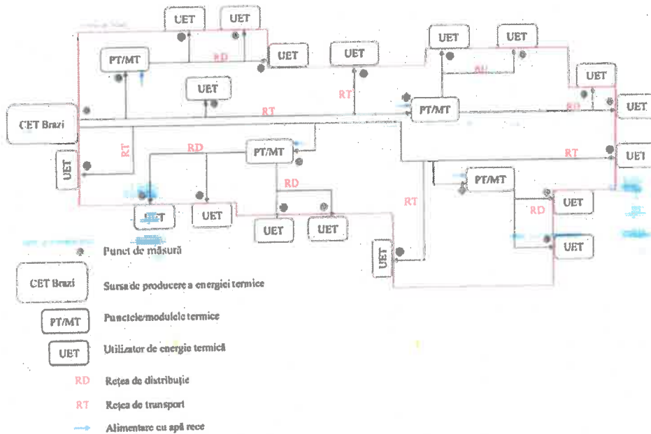
Figura 9.1 – Schema fluxului tehnologic din conturul de bilanț al RT și RD aferente PT/MT, cu punctele de măsură
