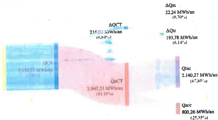
Figura 12.5 – Diagrama Sankey – bilanțul energetic real al RD CT – anul 2023
