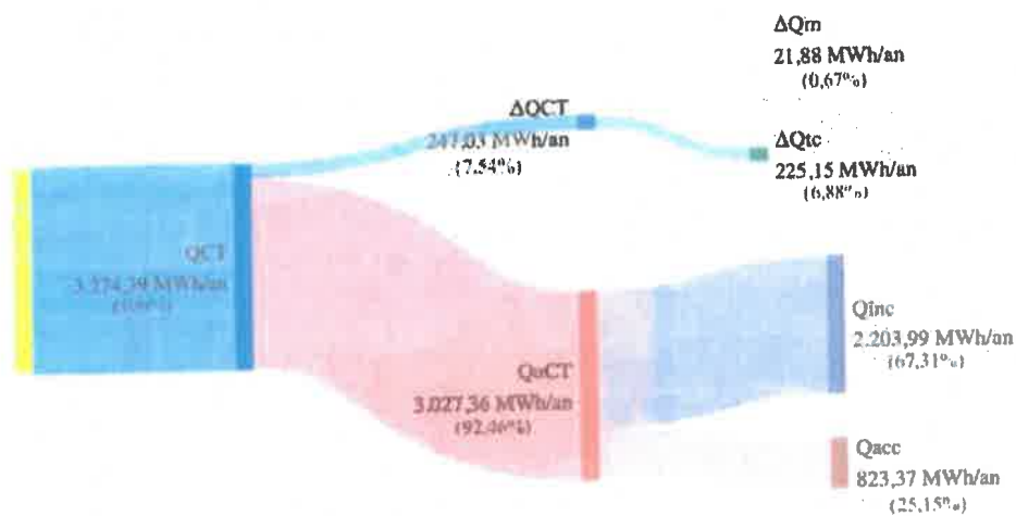
Figura 12.6 – Diagrama Sankey – bilanțul energetic real al RD CT – anul 2024
