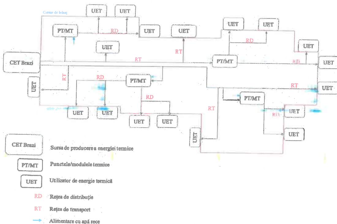
Figura 5.1 – Schema fluxului tehnologic din conturul de bilanț al RT și RD aferente PT/MT
