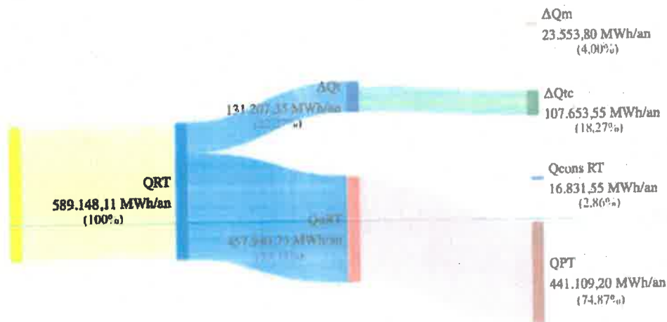
Figura 12.2 – Diagrama Sankey – bilanțul energetic real pentru RT – anul 2024
