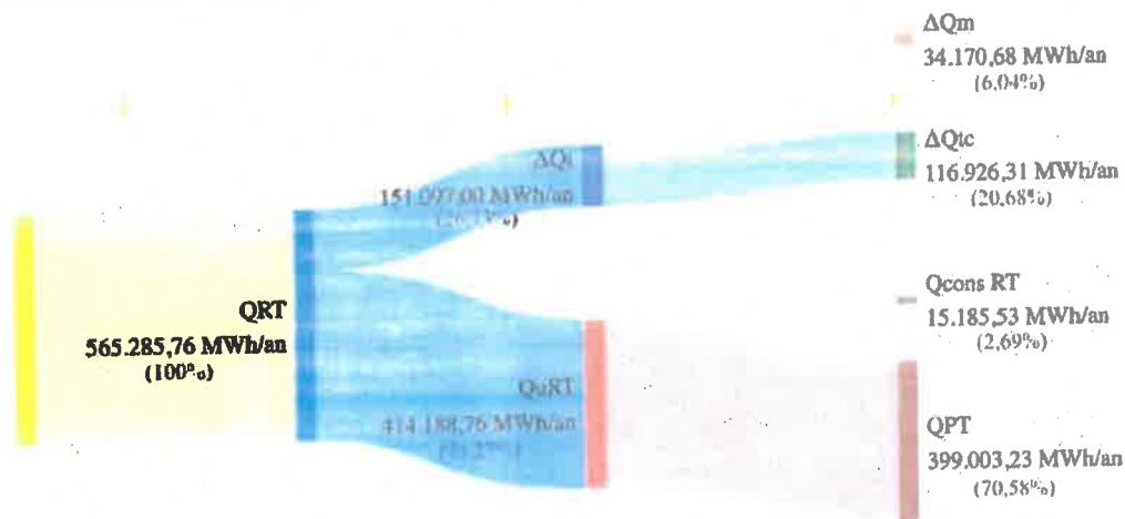
Figura 12.1 – Diagrama Sankey – bilanțul energetic real pentru RT – anul 2023
