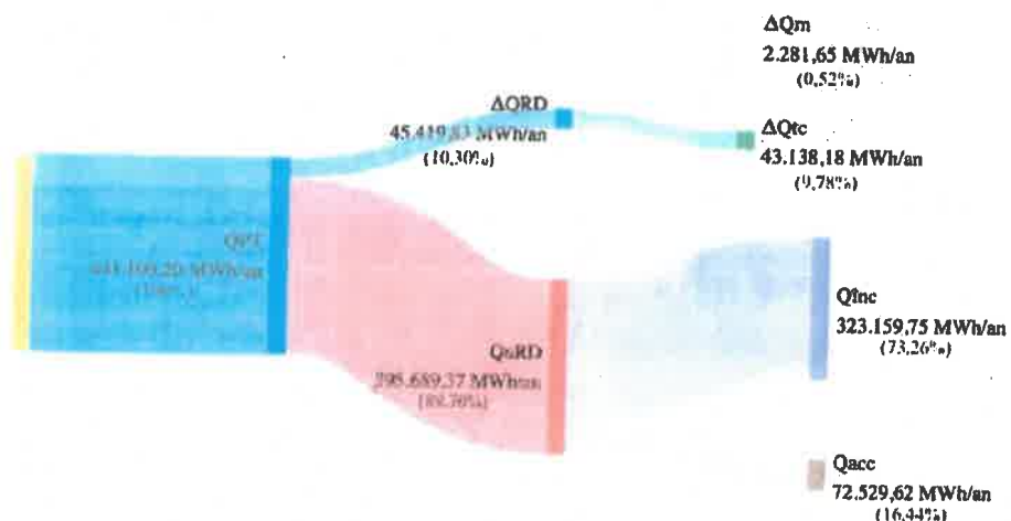
Figura 12.4 – Diagrama Sankey – bilanțul energetic real al RD PT/MT – anul 2024
